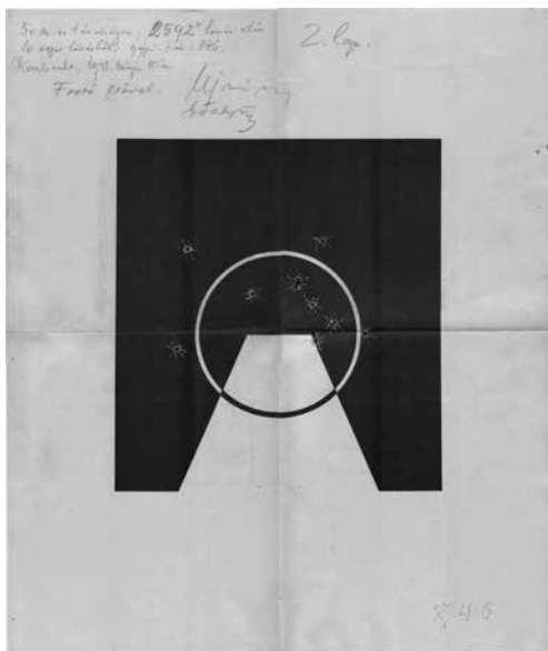
A tartóssági próba egyik lőlapja: tíz egyes lövés találati képe 50 m távolságon 2592 leadott lövés után (HL HM 36.409/eln. 3/a. oszt.– 1941)
