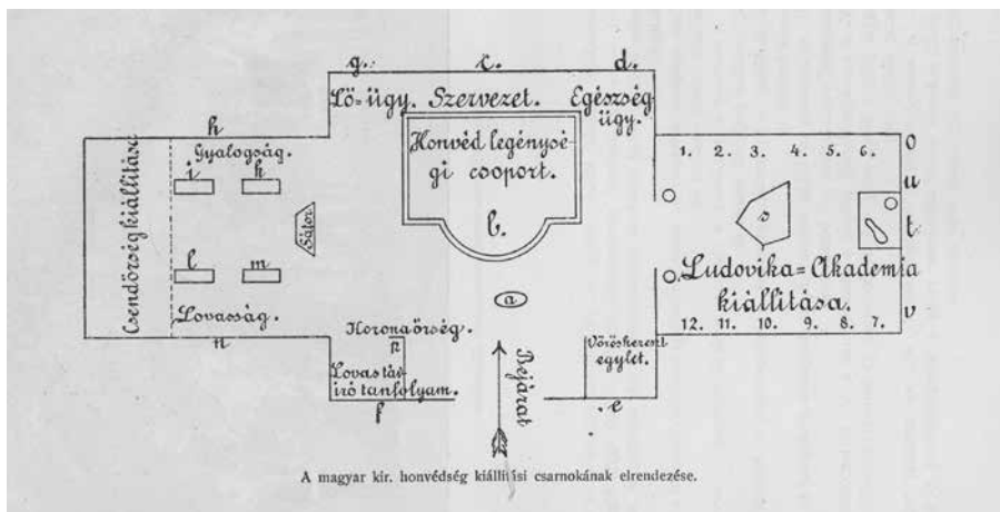
A honvédségi kiállítási pavilon alaprajza és tematikai elrendezése
