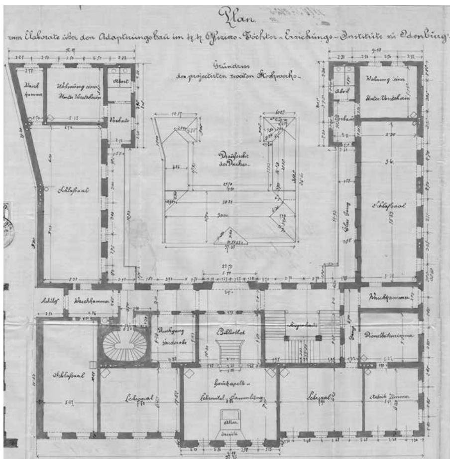
Az intézet tervrajza, 1883 (Forrás: MNL GYMSM SL APOe XXIV.8424)
