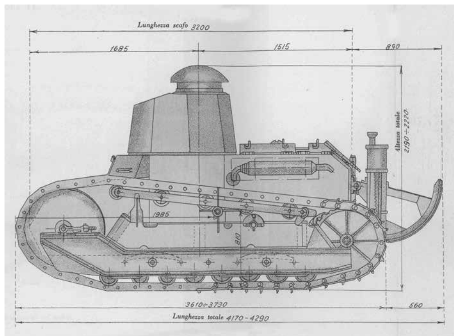
Fiat 3000B harckocsi. (Forrás: Istruzione sul carro armato Mod. 1921 e Mod. 1930. Roma, 1931. Tavola I.)
