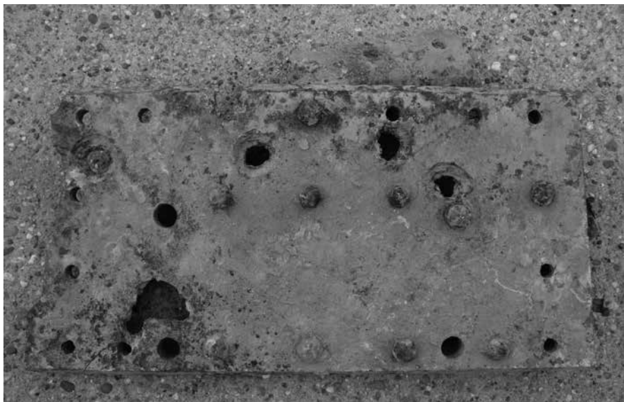
A páncéltorony orrlemeze kumulatív páncéltörő gránáttalálatok nyomaival (Ltsz.: 2015.6.1., Hadirégészeti Gyűjtemény)
