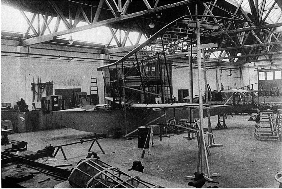
Lobner-féle repülőcsónak összeszerelése Albertfalván
