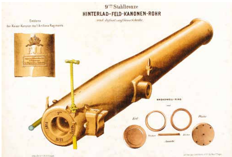
1875 M 9 cm táborigényű csőszerkezete
