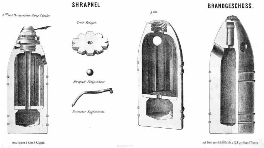
1875 M 8 cm srapnel és 9 cm gyújtólövedék metszete, középen srapnel töltelékgyöly és réz vezetőgyűrű ábrázolása
