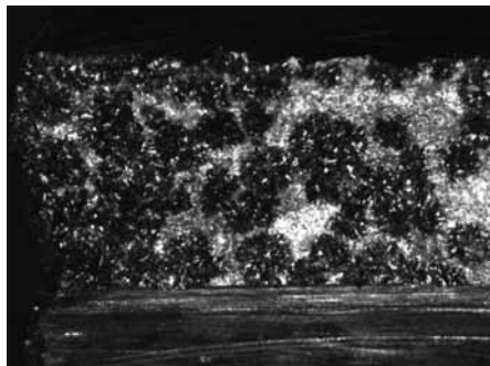
12. ábra. A repesz töretfelülete 8x-os nagyításban a belső felülethez közel
